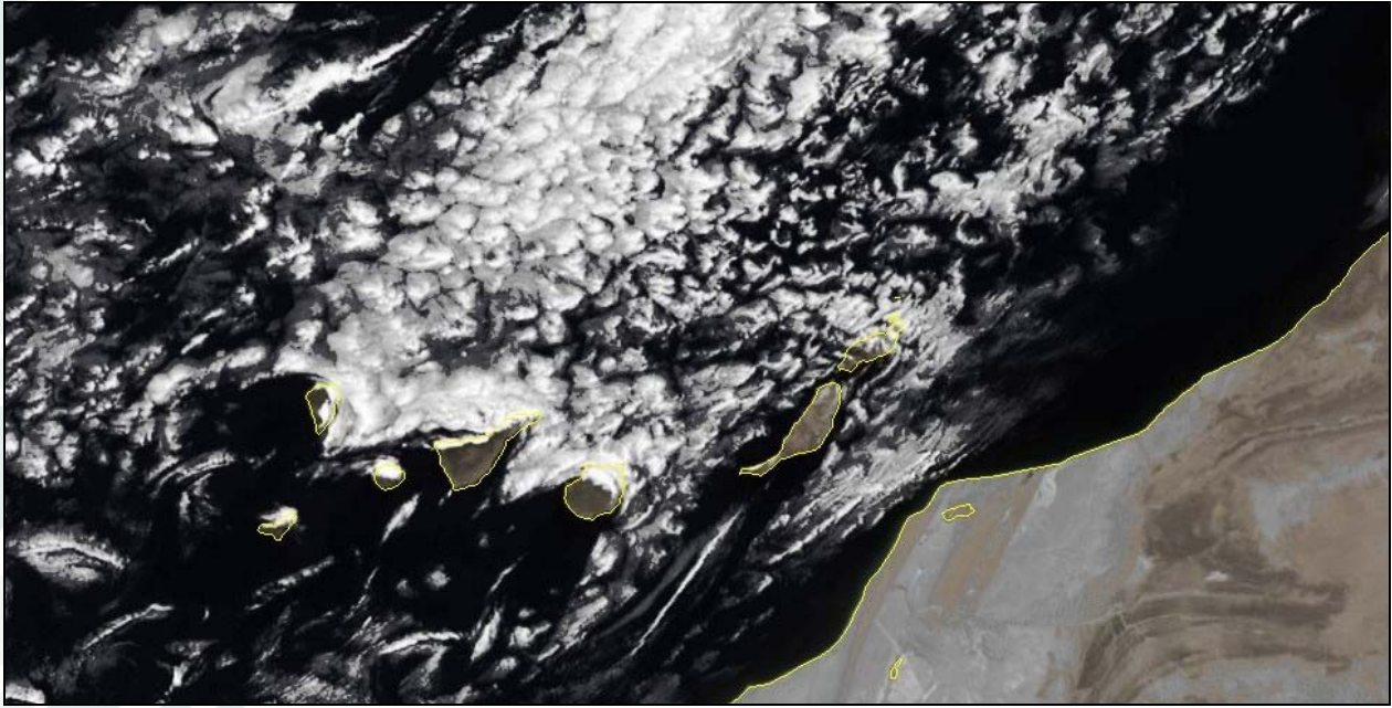
Imagen del satélite Meteosat 8 (visible): 21 de abril de 2009 a las 12 h UTC
