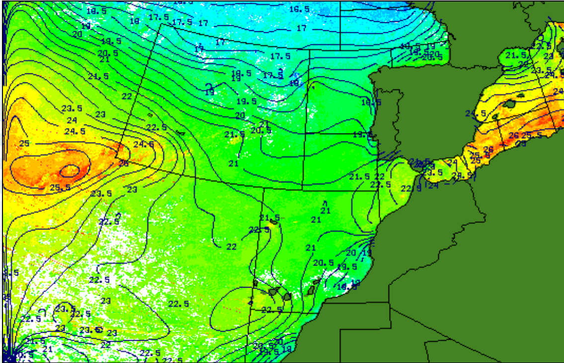
Temperaturas de la superficie del mar el 7 de julio de 2007 (INM)
