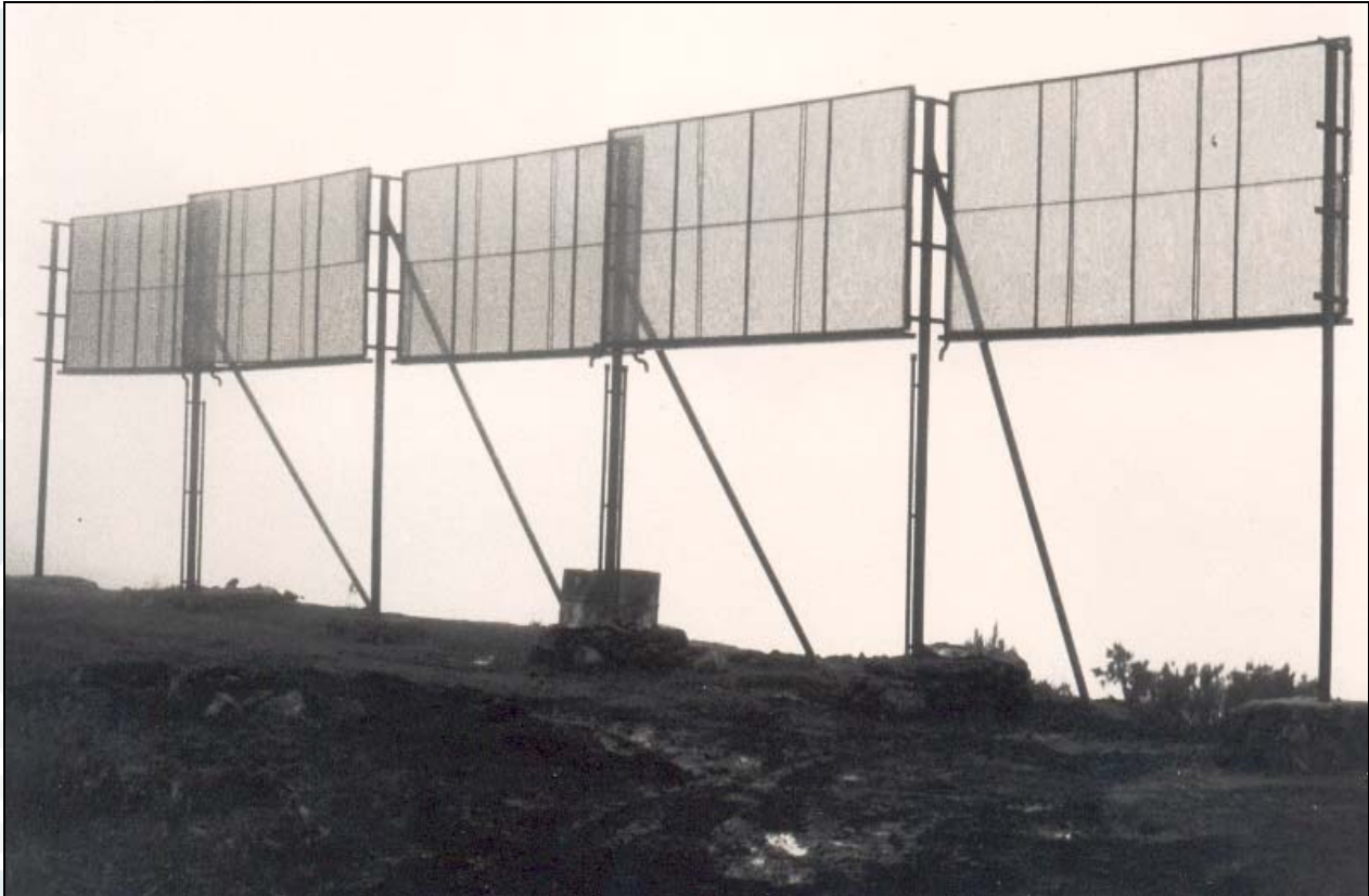
Captaniebla rectangular de 40 m 2 colocado en la Hilera – Cumbre Nueva (La Palma - 1987) a 1350 m.
