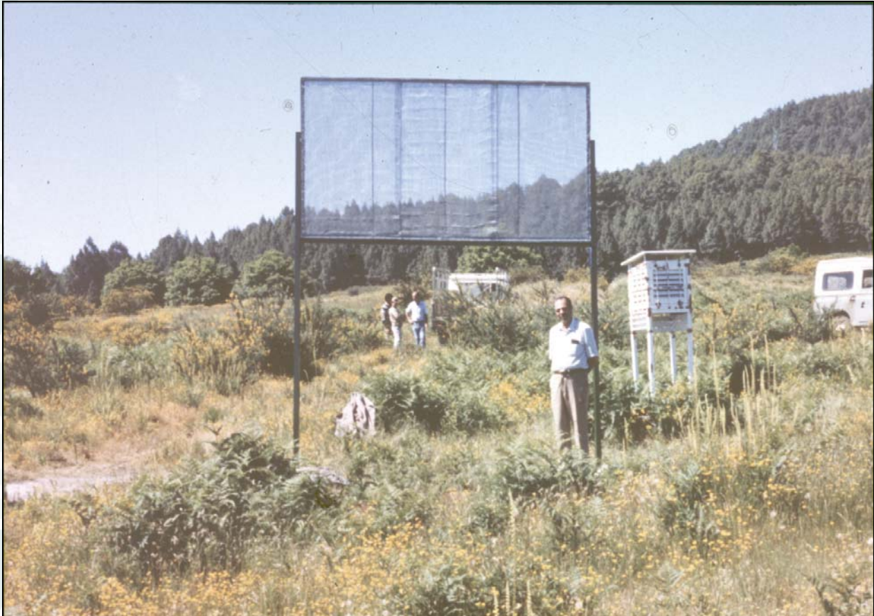
Captanieblas rectangular de 3* 1.5m 2 fabricado en las instalaciones del ICONA
