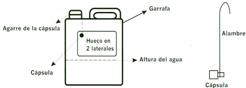
Figura 43.- Componentes de trampa de agua para polilla guatemalteca
