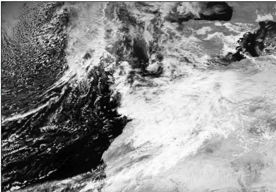
Imagen del satélite Meteosat 8 (visible): 24 de enero a las 12 h UTC
